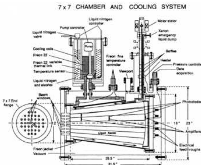
FIG. 70 Schematic of the MIT-ITEP-Dubna LXe scintillation calorimeter prototype (4).
